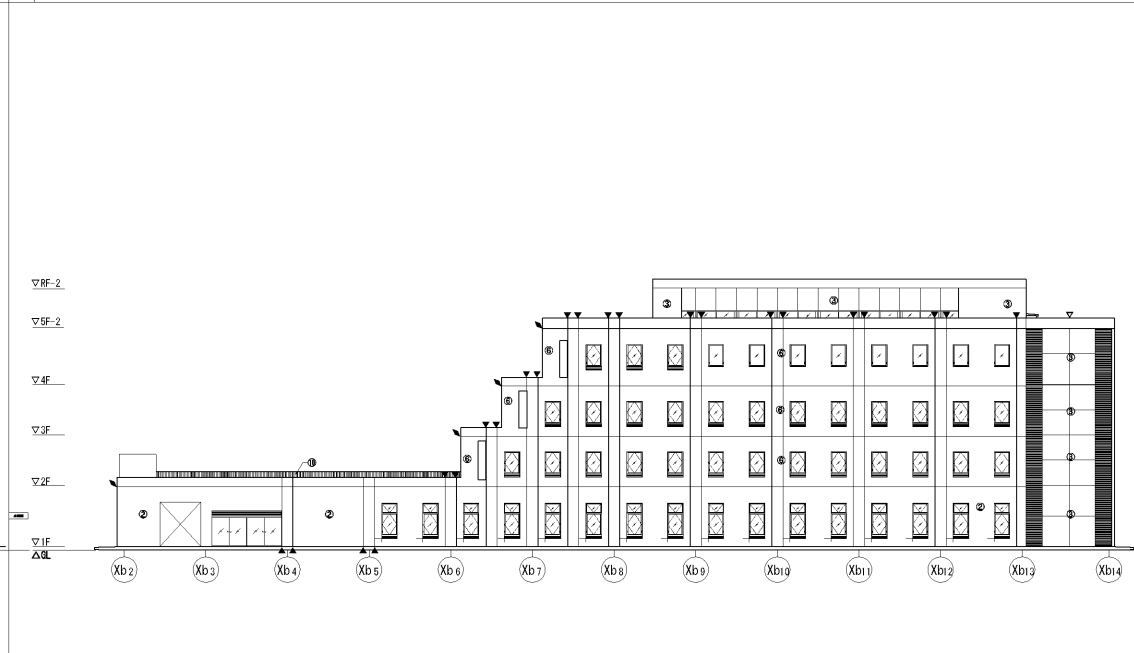
4 議会棟 北側立面図
