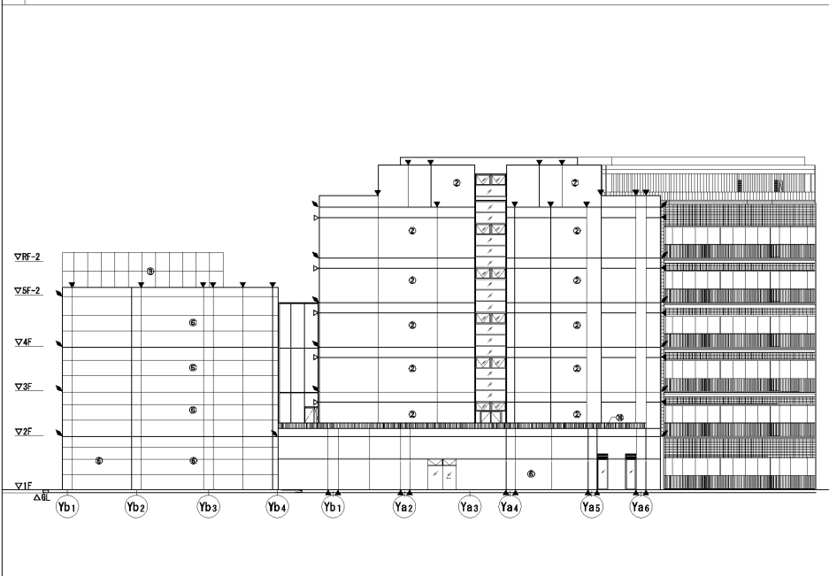
3 東側立面図
