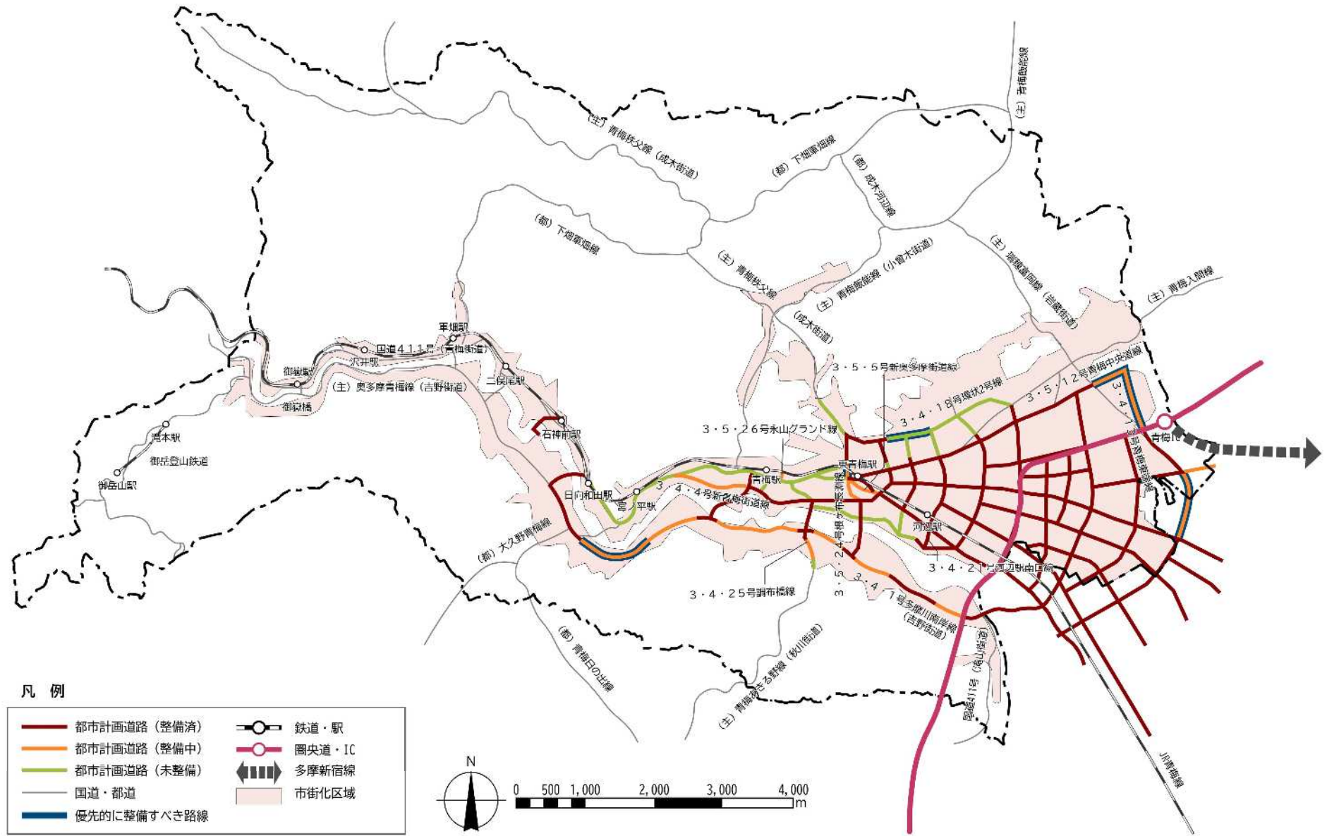
図 交通体系の整備方針図(2) (幹線道路の整備計画図)
