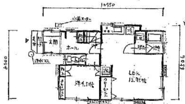
1F平面図
