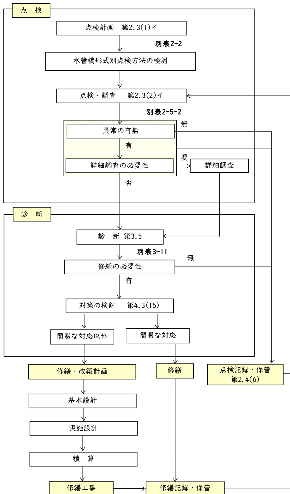
(別表3-12) 水管橋の診断フロー
