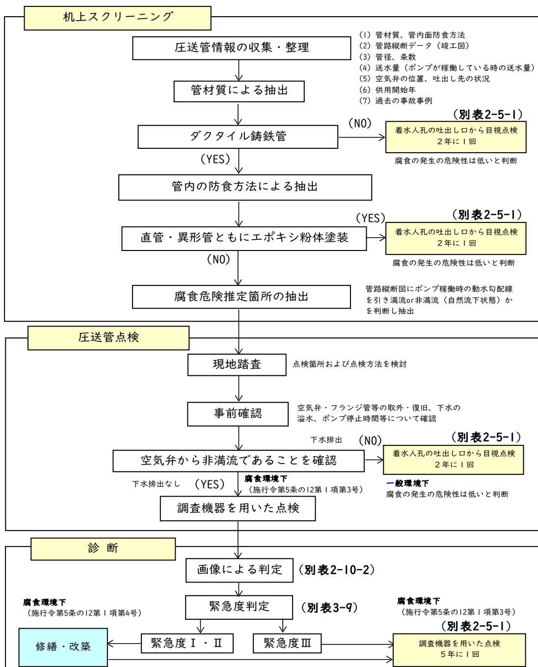
(別表3-10) 圧送管の診断フロー
