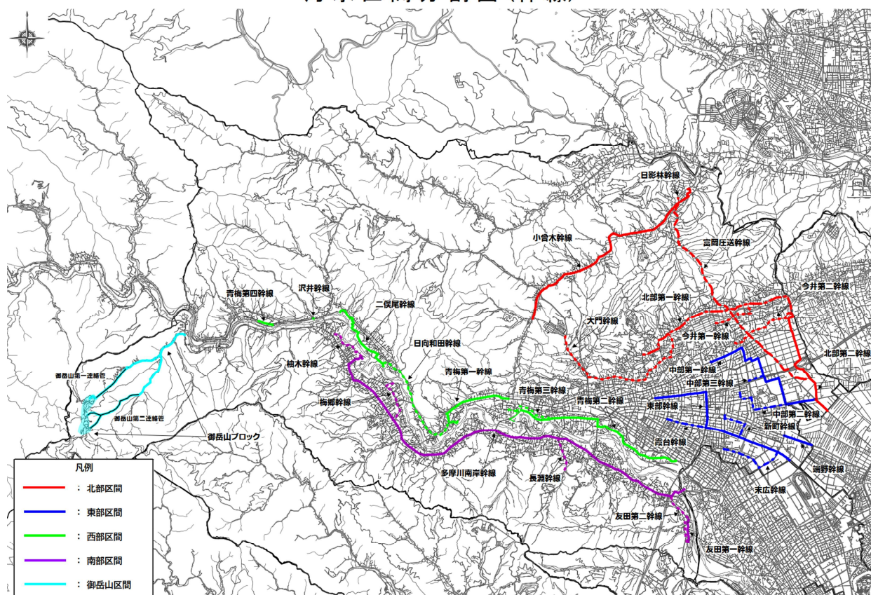
汚水区間分割図(幹線)
