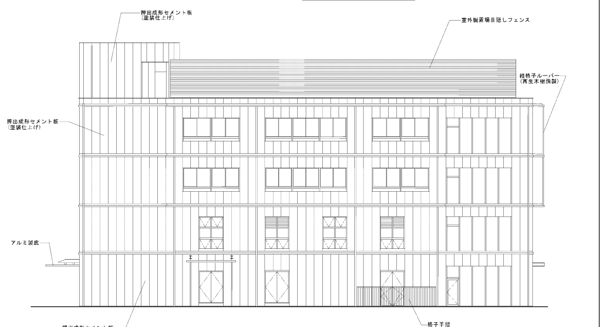
西側立面図
