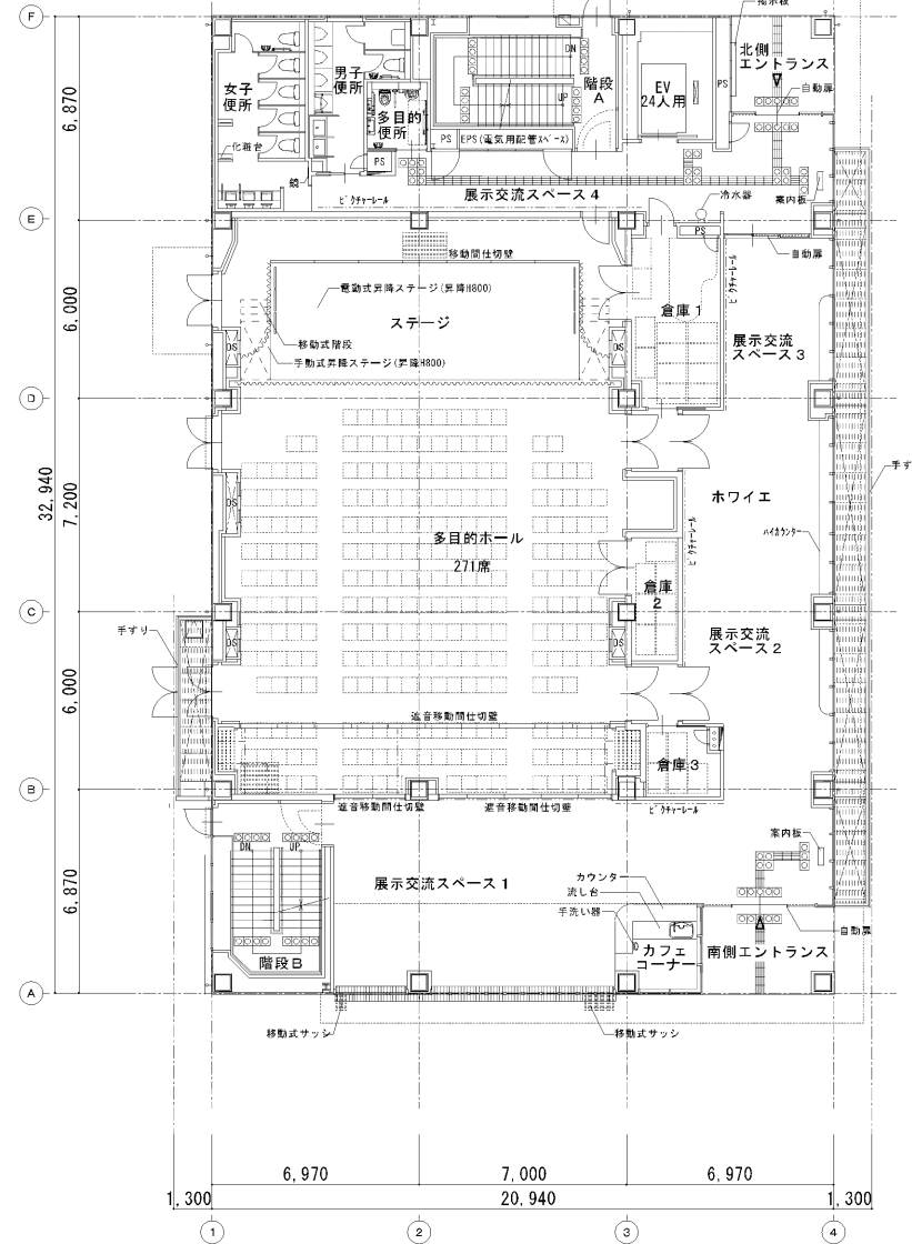
1階平面図
