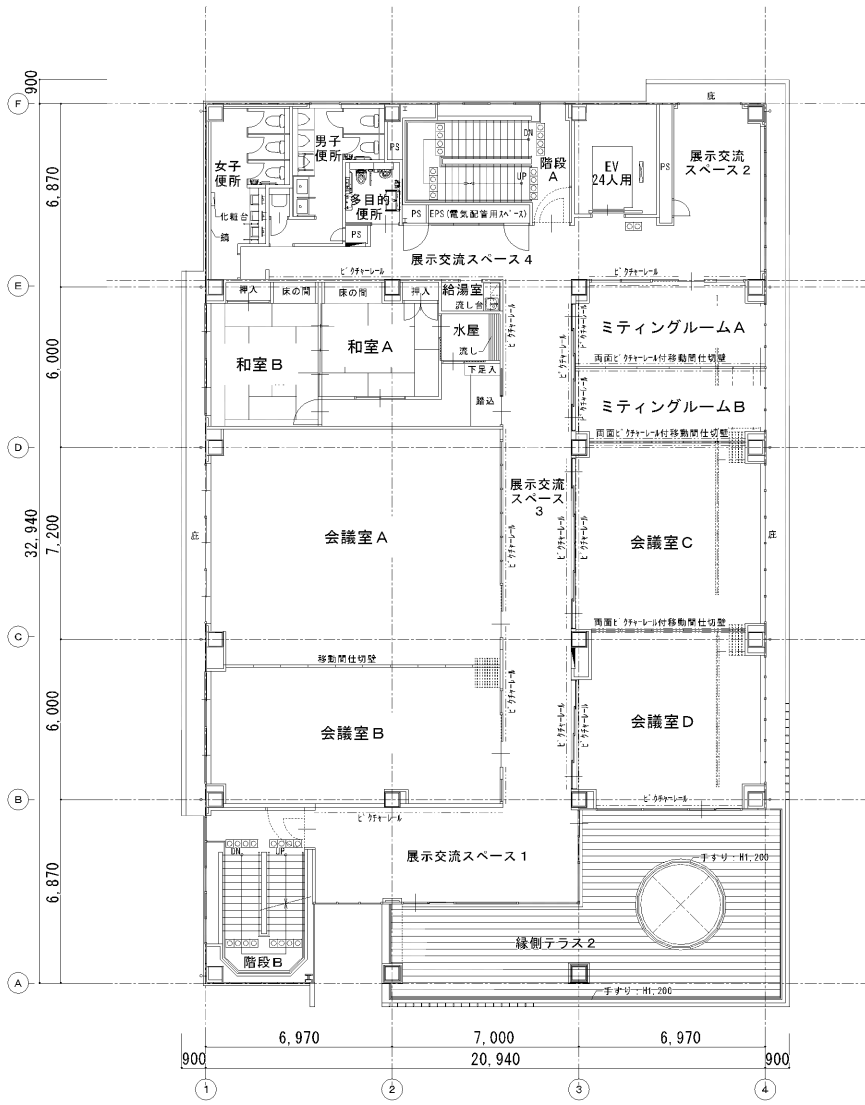
4階平面図
