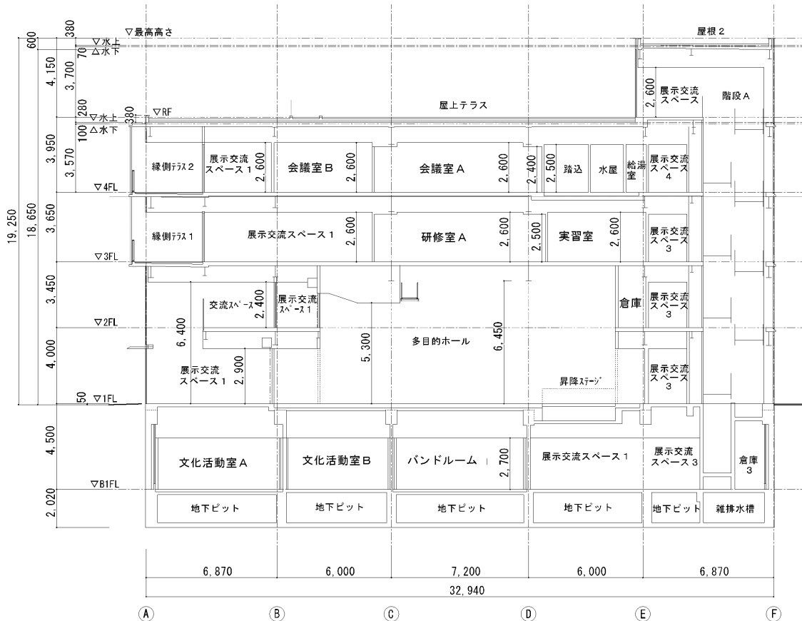
A~A' 断面図 (南北断面図)
