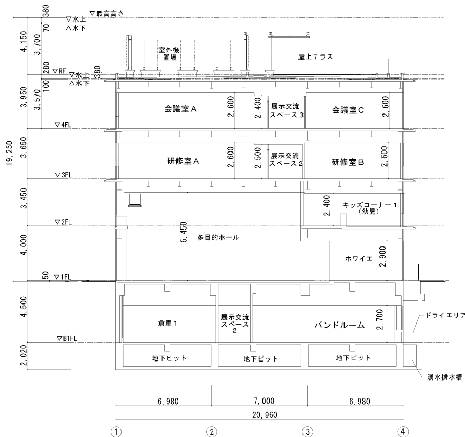
B~B' 断面図 (東西断面図)
