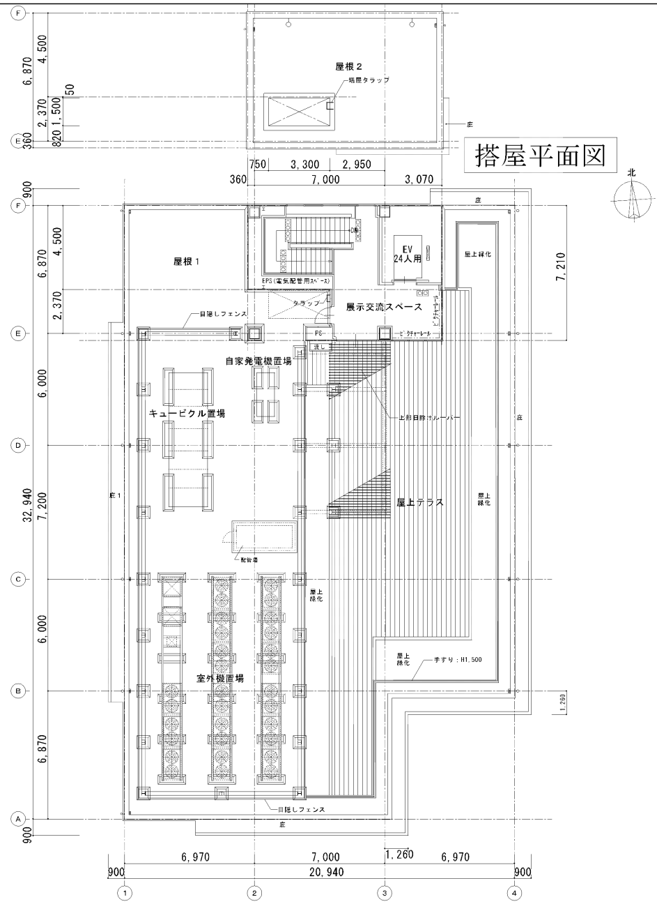
屋上平面図
